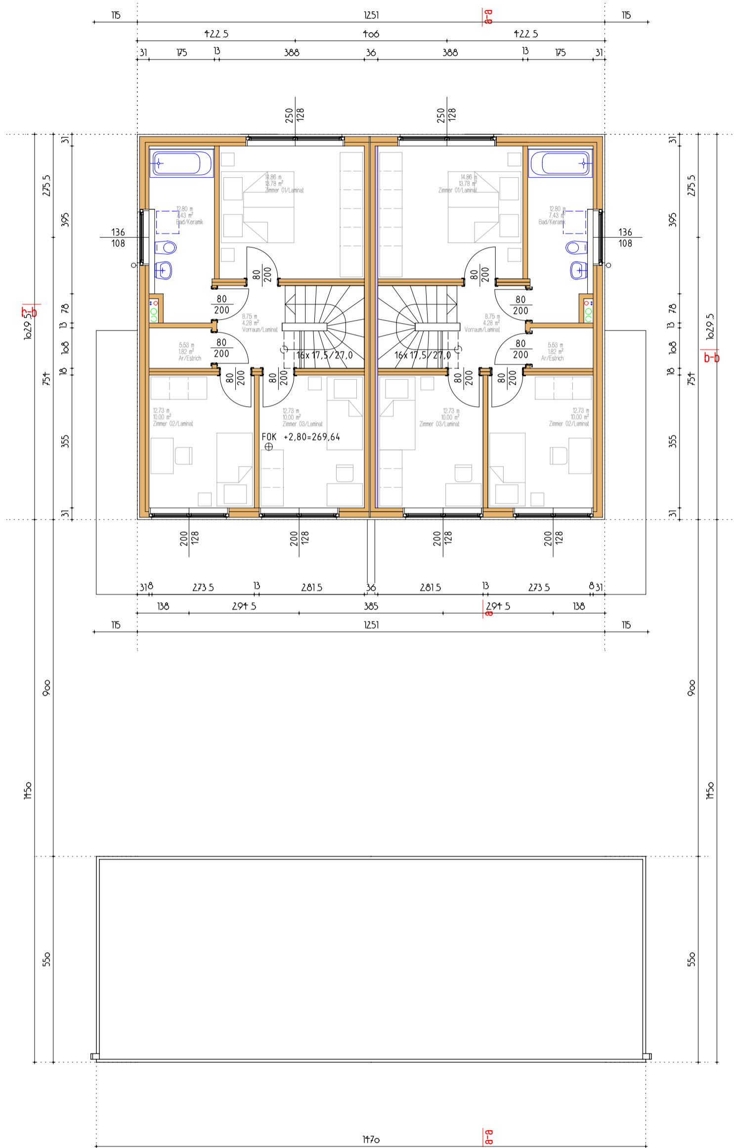
Obergeschoss 1/100
