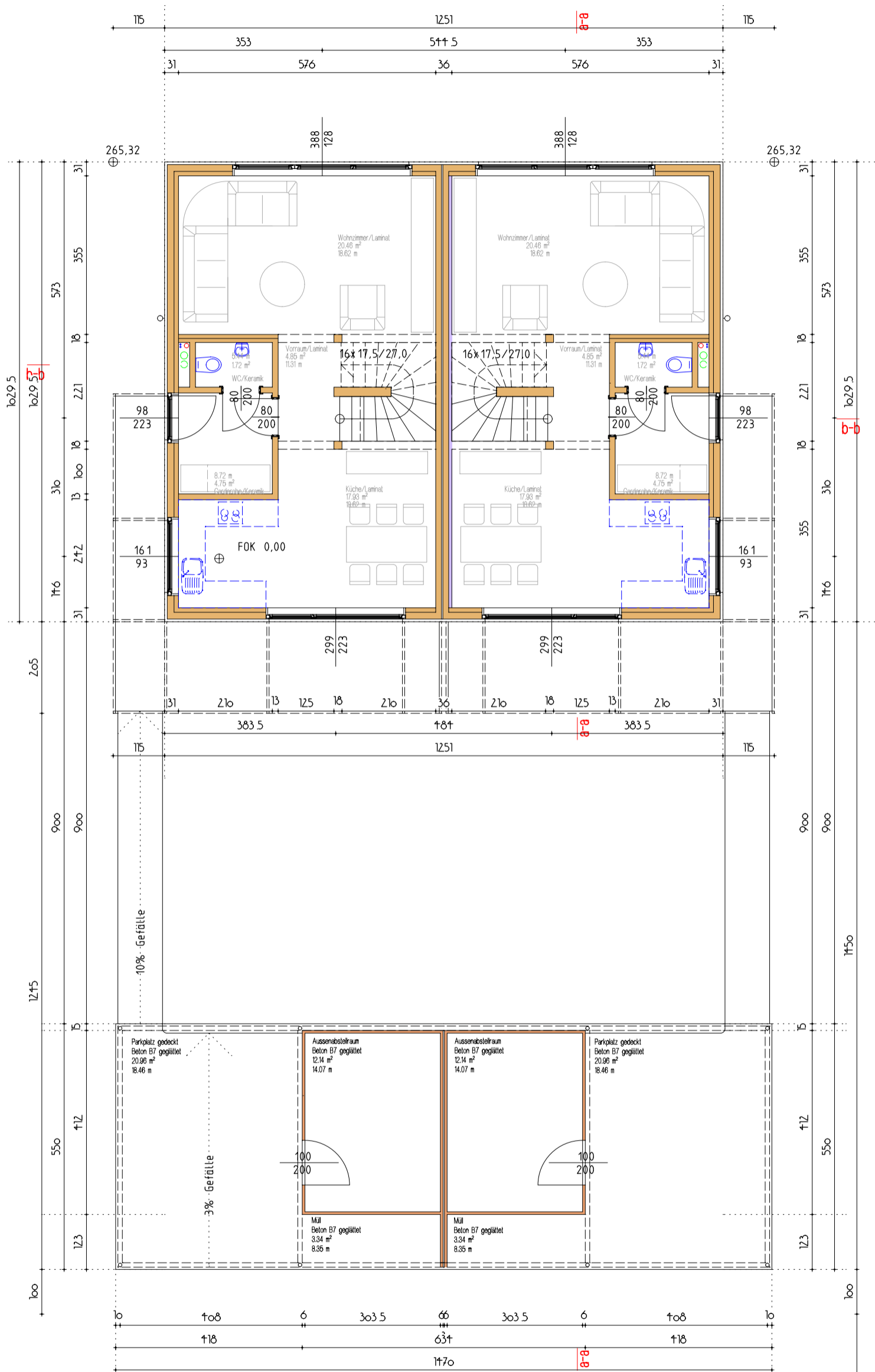
Erdgeschoss 1/100
