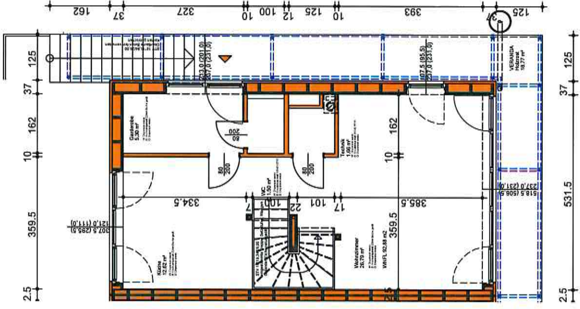
ERDGESCHOSS
