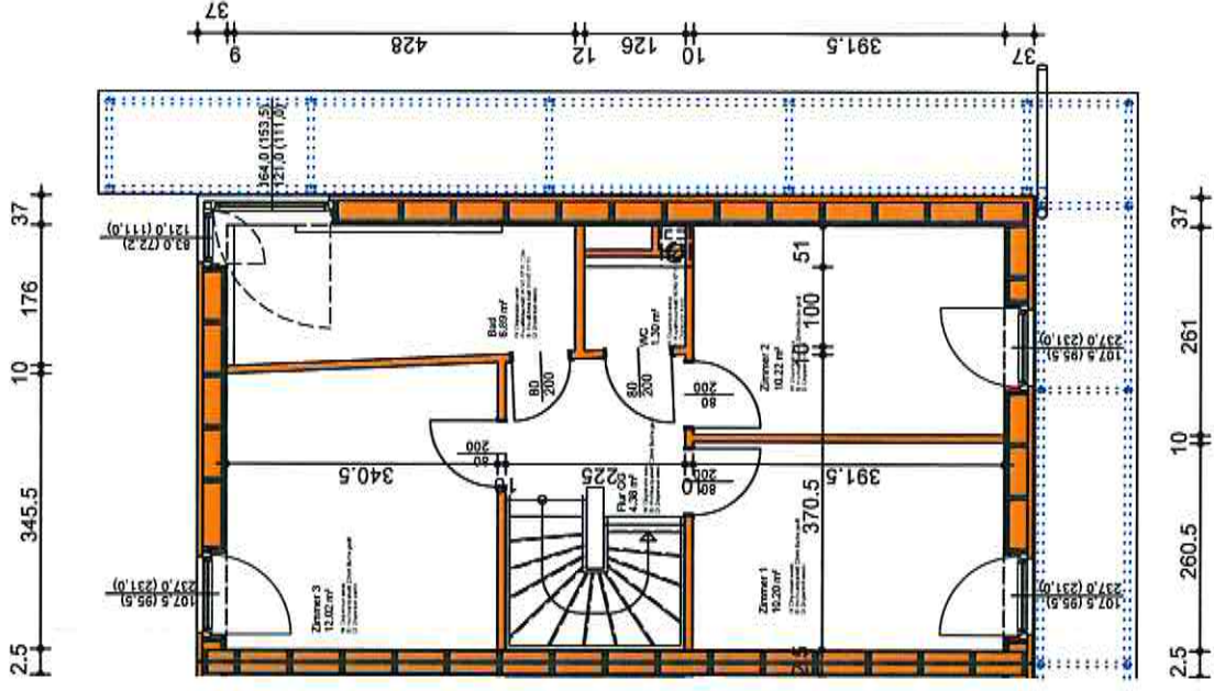
OBERGEHOSS
