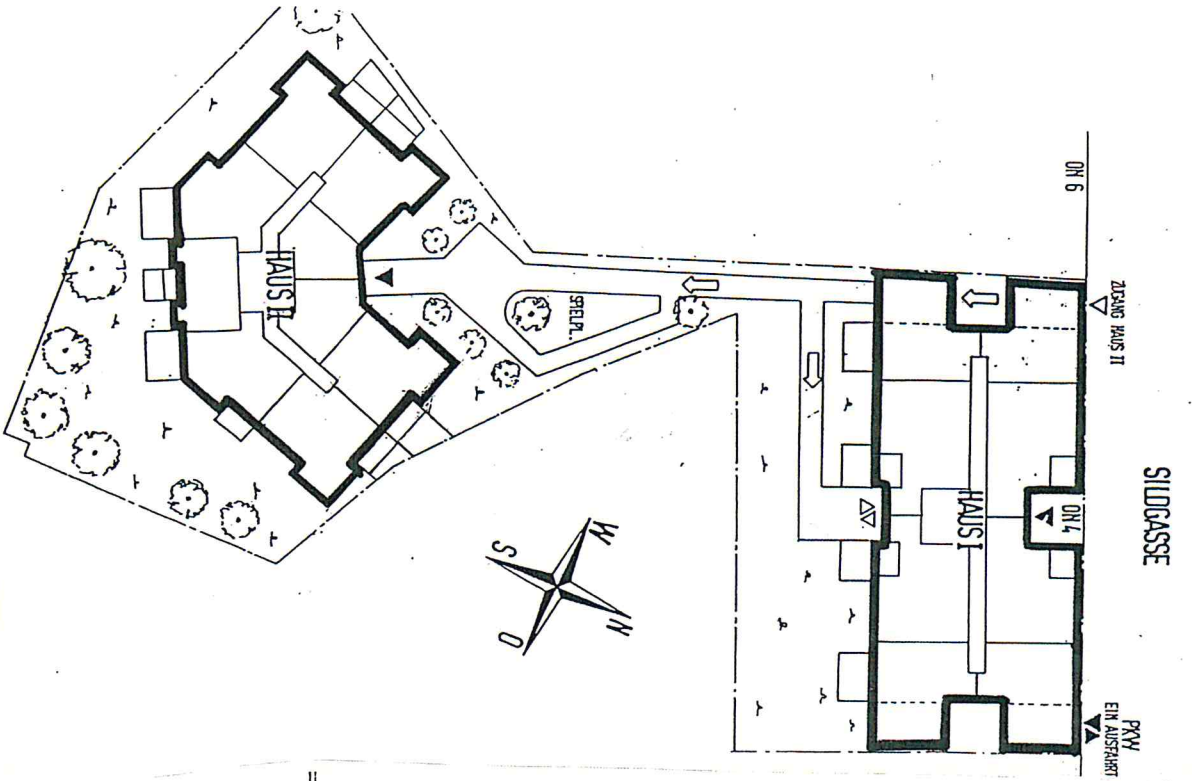
1210, SILDG. 4 LAGEPLAN 1:500 ÜBERSICHT ZUR ANORDNUNG DER WOHNUNGEN
